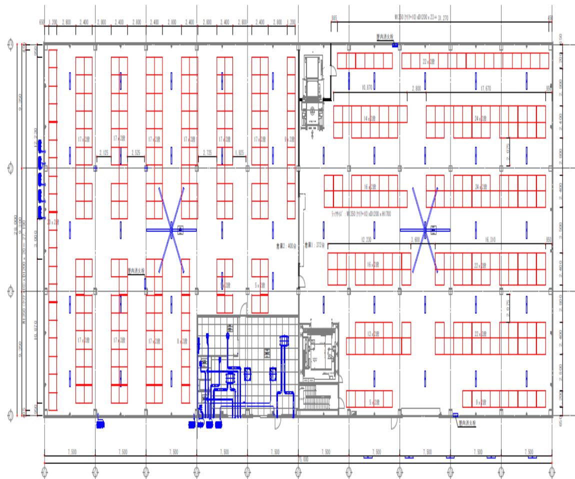
1階平面図 S-1/250
